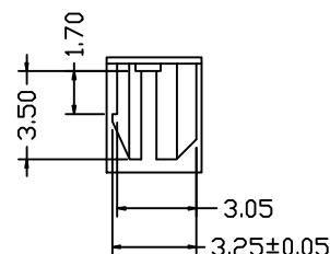
DETAIL A 2:1
